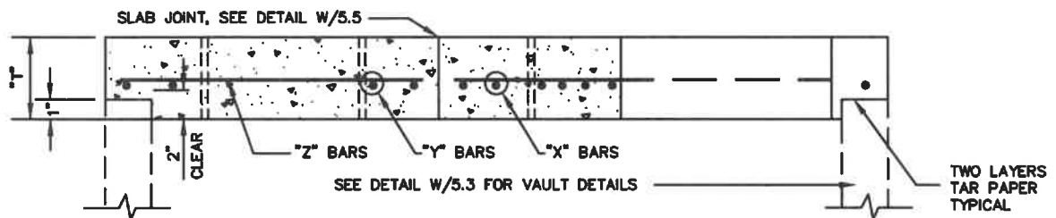
SECTION A-A
