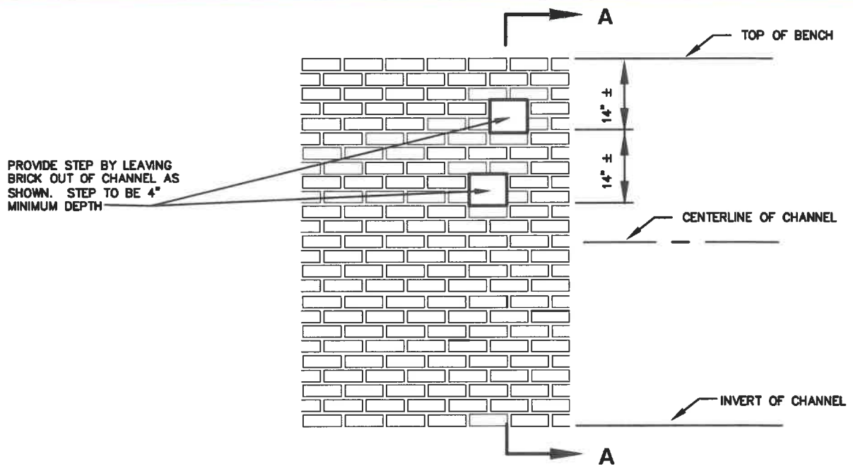
ELEVATION
